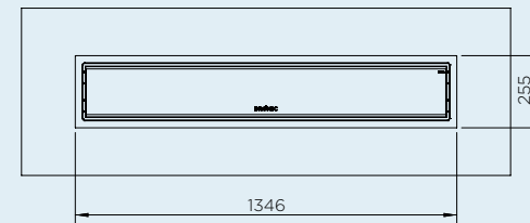
CAVIDAD MÍNIMA OPCIÓN 2
