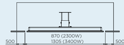
CAVIDAD MÍNIMA OPCIÓN 1
