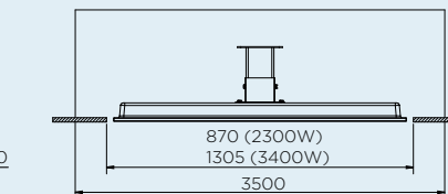
CAVIDAD MÍNIMA OPCIÓN 2
